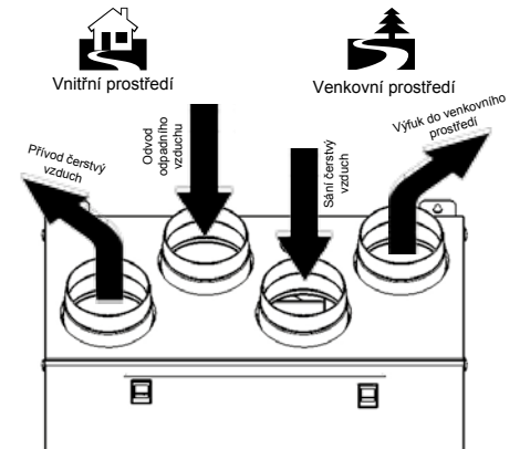
Obr. 3.b Připojení při PRAVÉM provedení
