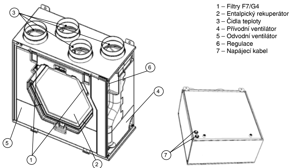
Obr. 8.a Vnitřní komponenty
